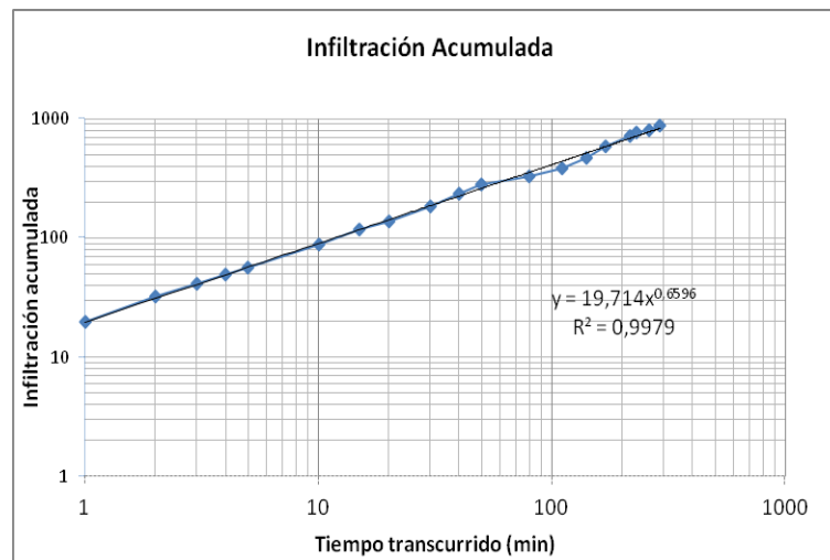
Gráfico 2: Infiltración acumulada
